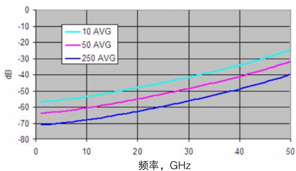
80E10 插入损耗(S21)动态范围
