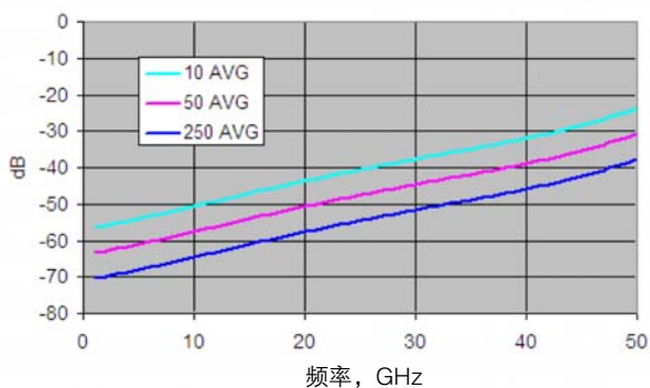
80E10 回波损耗(S11)动态范围
