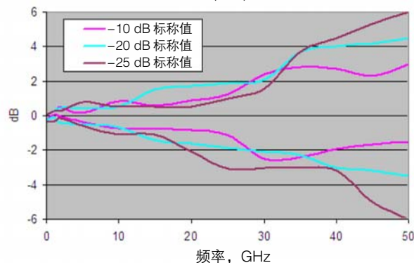
80E10 回波损耗(S11)幅度不确定性
