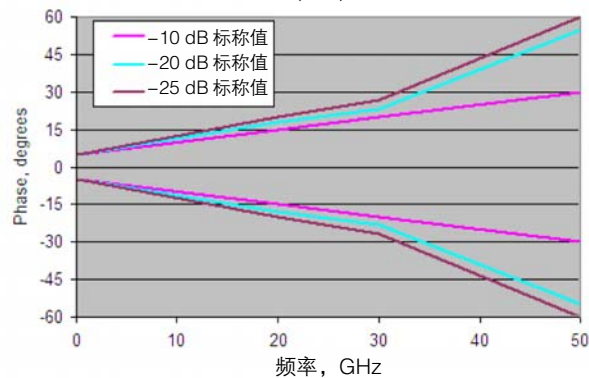
80E10 回波损耗(S11)相位不确定性
